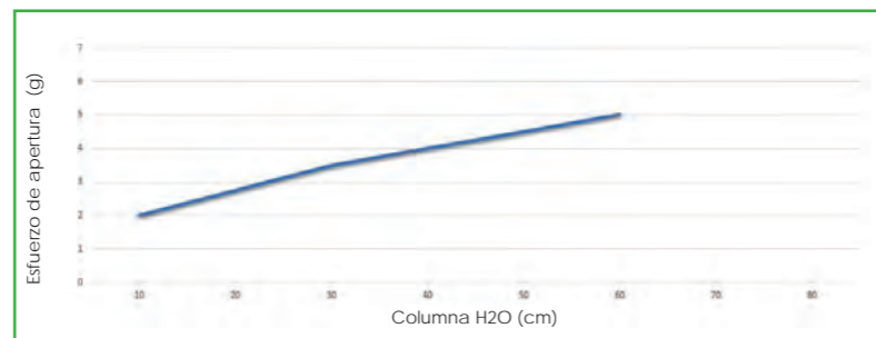
Esfuerzo de apertura, +-15% Art. 4006i
