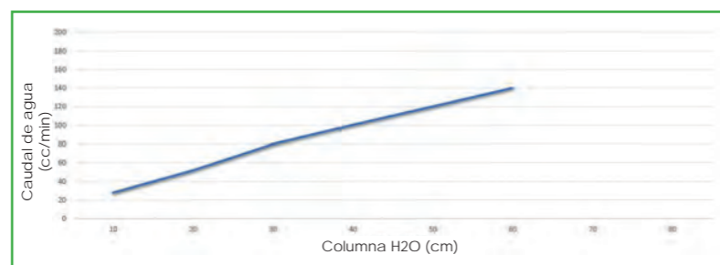
Caudal de agua, +-15% Art. 4006i
