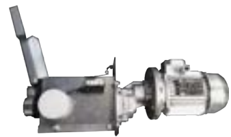
4473T3/4SC Gruppo traino con motore trifasico 0,75 KW per sensore capacitivo
