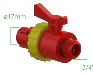
4778D Rubinetto a sfera 3/4" per tubo ø 12x17mm con ghiera
