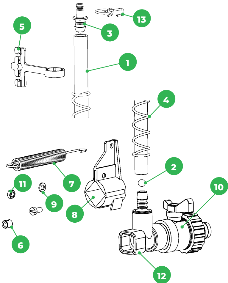
4957N Kit finelinea per tubo quadro h: 500mm, ø12 4957F versione flushing con art.4773 P
