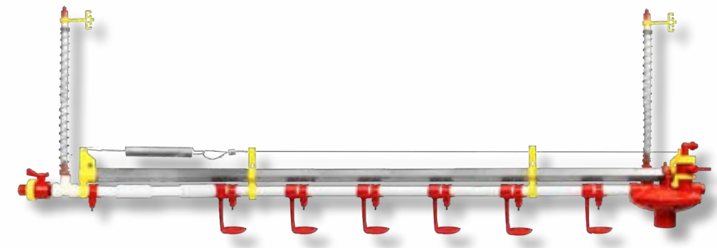
Linea abbeveraggio tubo tondo ø 26,6 mm
