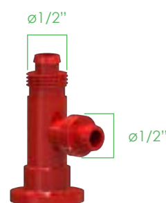
4771T Connessione a T tubo flex o spirale øint12,5x15mm
