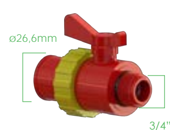
4785 Rubinetto a sfera 3/4" M con raccordo a tubo tondo ø26,6mm
