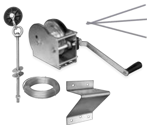
4860F Kit sollevamento linee di alimentazione. Con uso di argani e pulegge è assicurato il rapido sollevamento delle linee, permettendo un facile accesso all'area dell'allevamento durante le operazioni di manutenzione e pulizia. Il cavo può essere posizionato in modo la lavorare in ogni direzione, grazie alla particolare conformazione della puleggia ø90mm.
